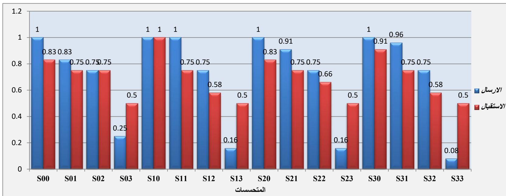
الشكل (٦) مخطط يوضح معدل إرسال واستقبال البيانات لكل مستشعر بالشبكة المقترحة
