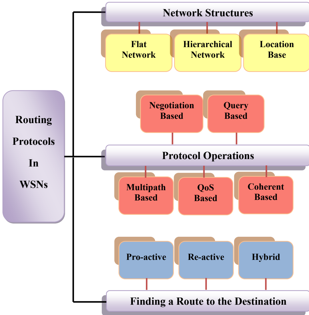
الشكل (٢) تصنيفات أنواع بروتوكولات التوجيه في شبكات الاستشعار اللاسلكية
