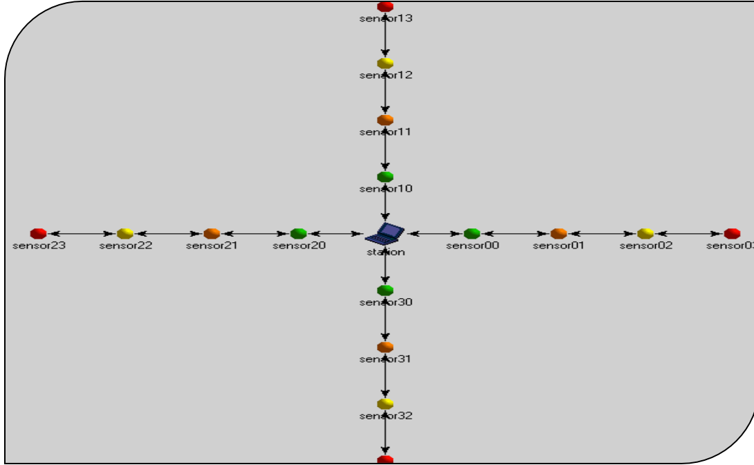
الشكل (٣) شبكة الاستشعار اللاسلكية المقترحة لخلق تقاطع مرور ذكي.
